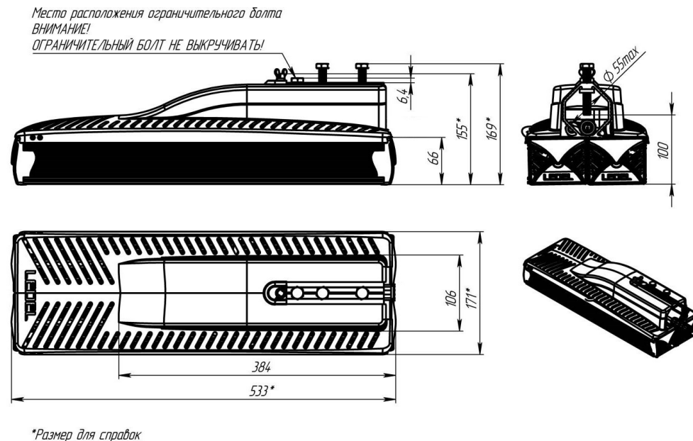
Рисунок 1 Габаритные размеры светильника «L-street 48»
